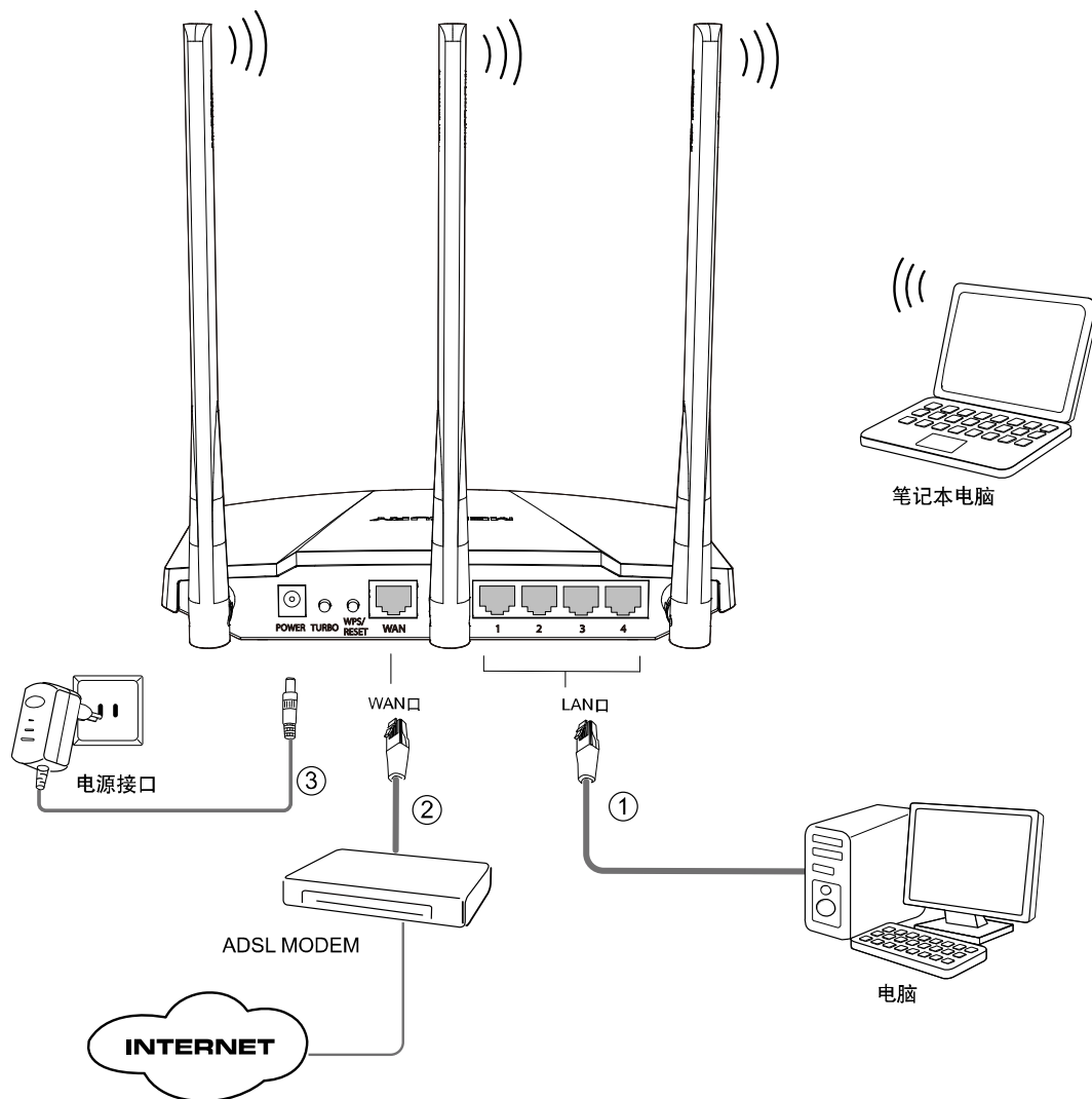
图2-3 硬件连接图
