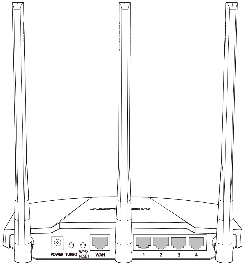
图2-2 MW316R 后面板示意图
