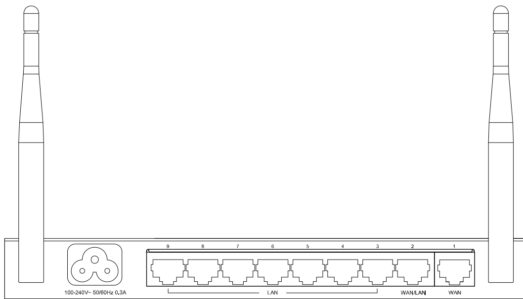
图 2-5 MR308VPN后面板示意图
