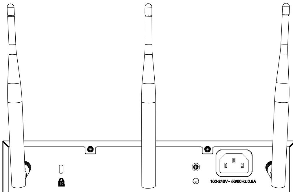
图 2-6 MR450VPN后面板示意图
