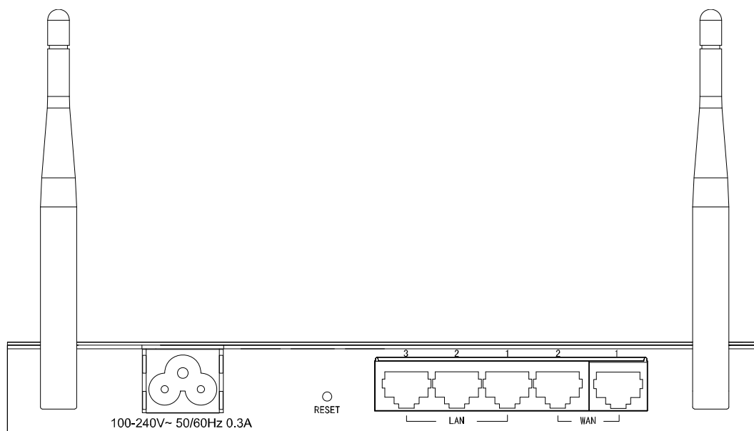
图 2-4 MR300VPN后面板示意图
