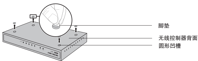
图3-1 桌面安装示意图
