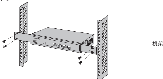
图3-3 机架安装示意图
