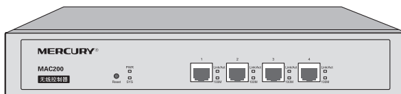
图2-3 MAC200前面板示意图
