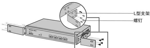
图3-2 支架安装示意图
