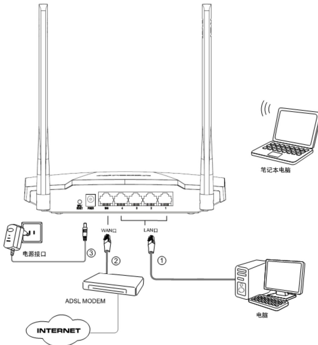
图 2-3 硬件连接图
