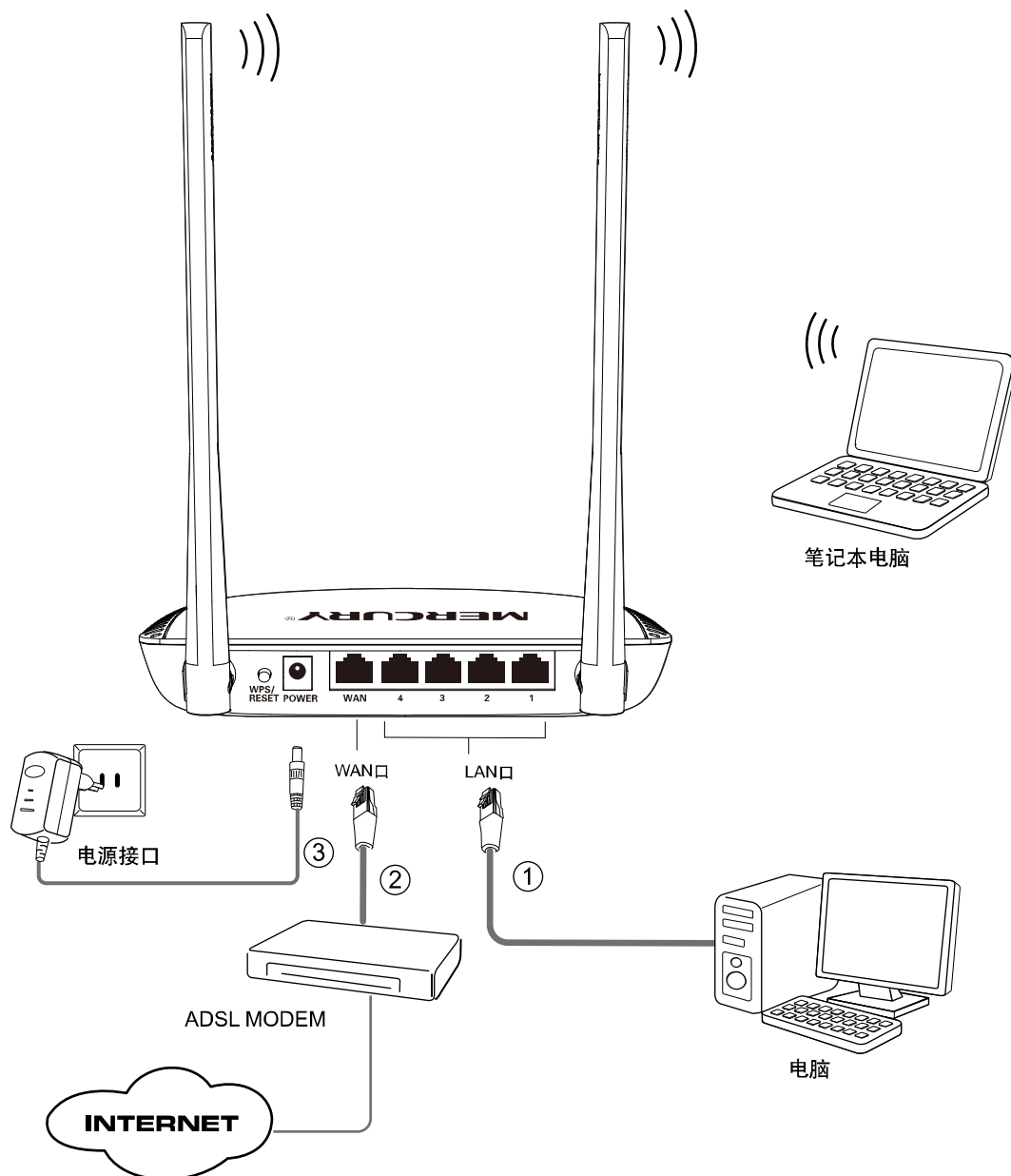
图2-3 硬件连接图
