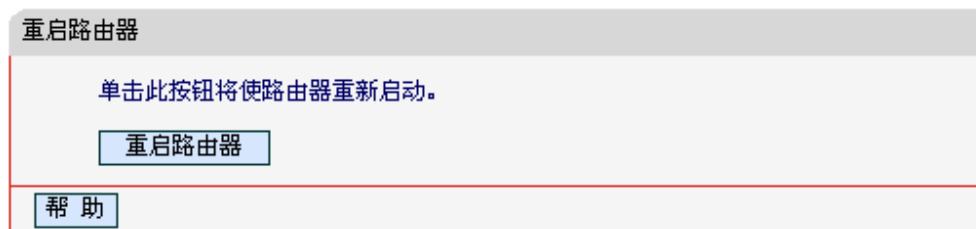
图4-65 重启路由器
