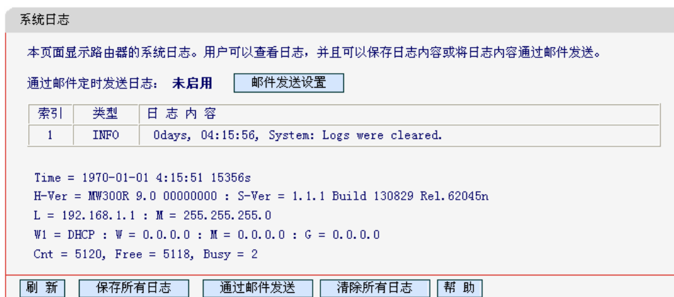
图4-67 系统日志
