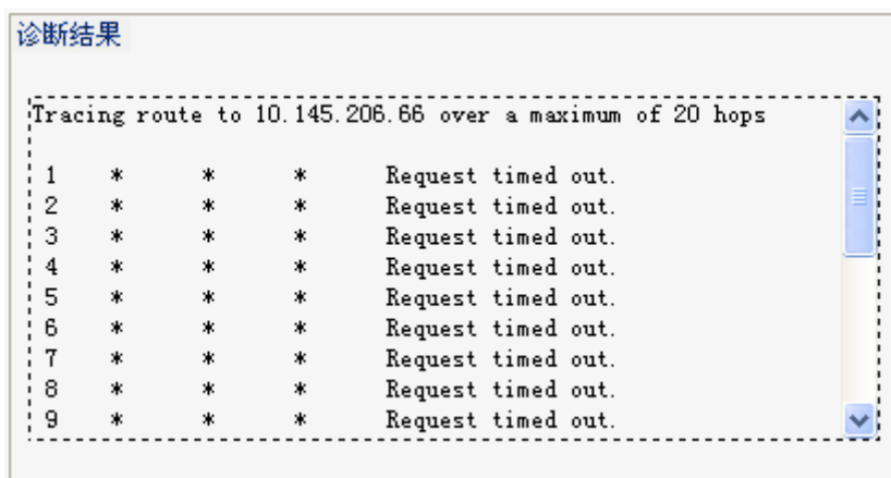
图4-59 Tracert 诊断结果—失败
