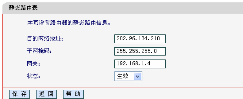
图4-46 添加静态路由条目
