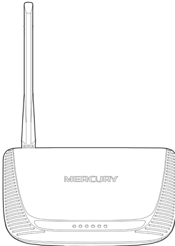
图 3-1 MW150R 前面板示意图
