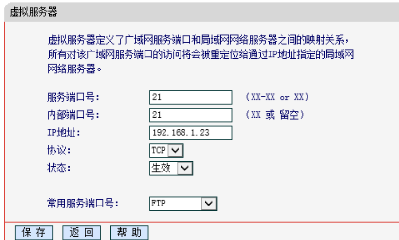
图 5-24 设置虚拟服务器条目
