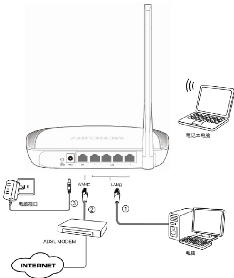
图 4-1 MW150R 硬件安装示意图
