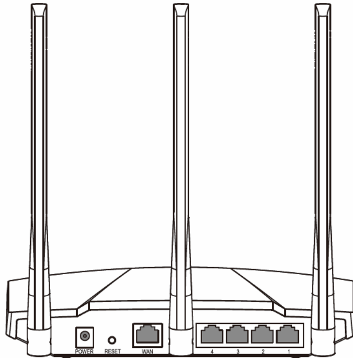
图 2-2 MW450R 后面板示意图
