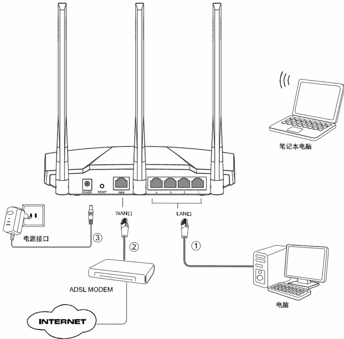
图 2-3 硬件连接图
