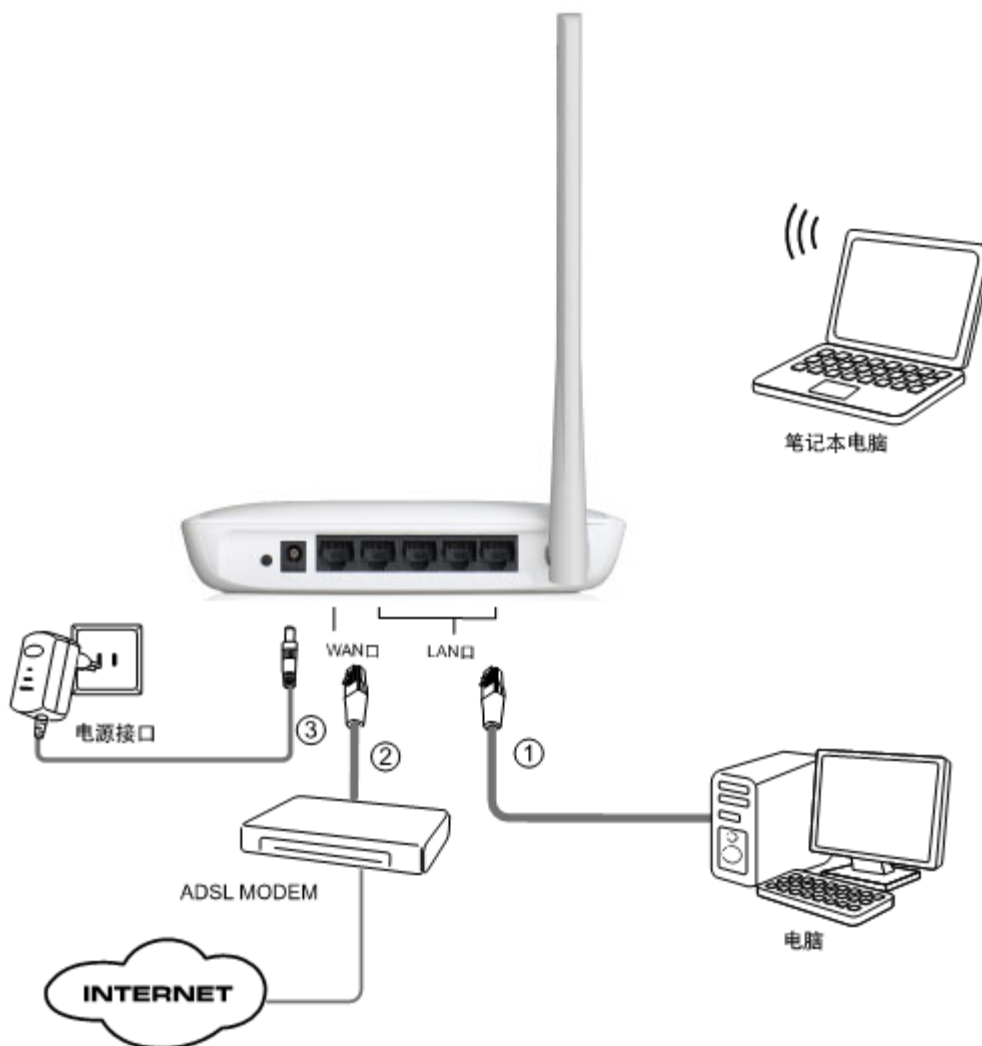
图 4-1 MW150R 硬件安装示意图
