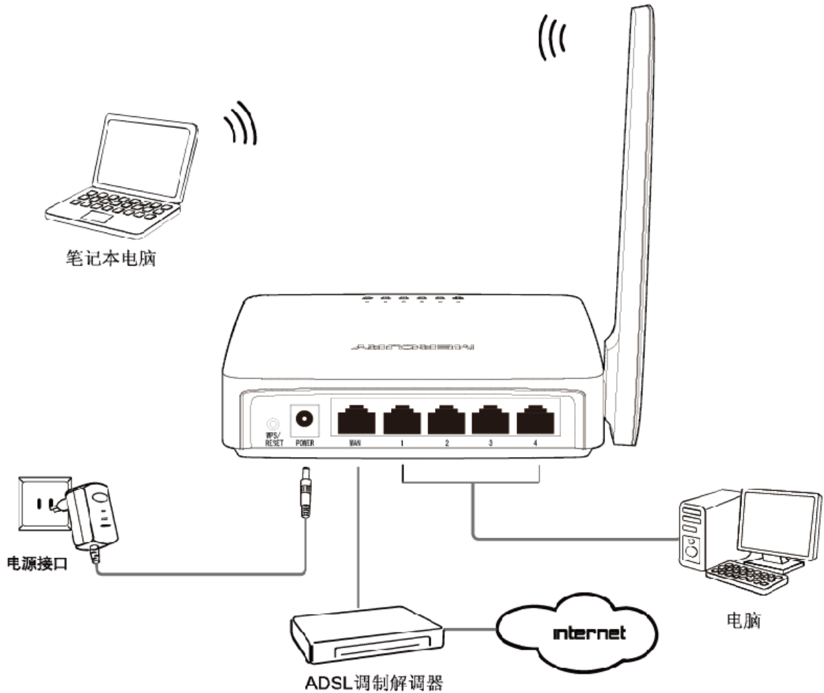
图 2-3 硬件连接图
