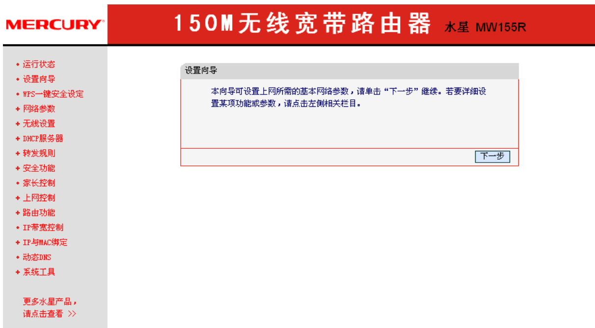
图 3-4 设置向导
