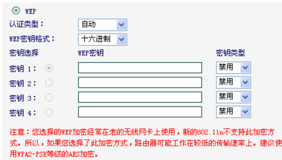
图 4-14 WEP 加密
