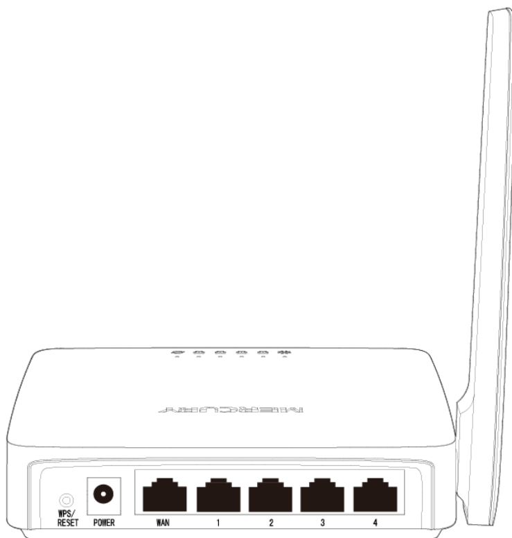
图 2-2 MW155R 后面板示意图
