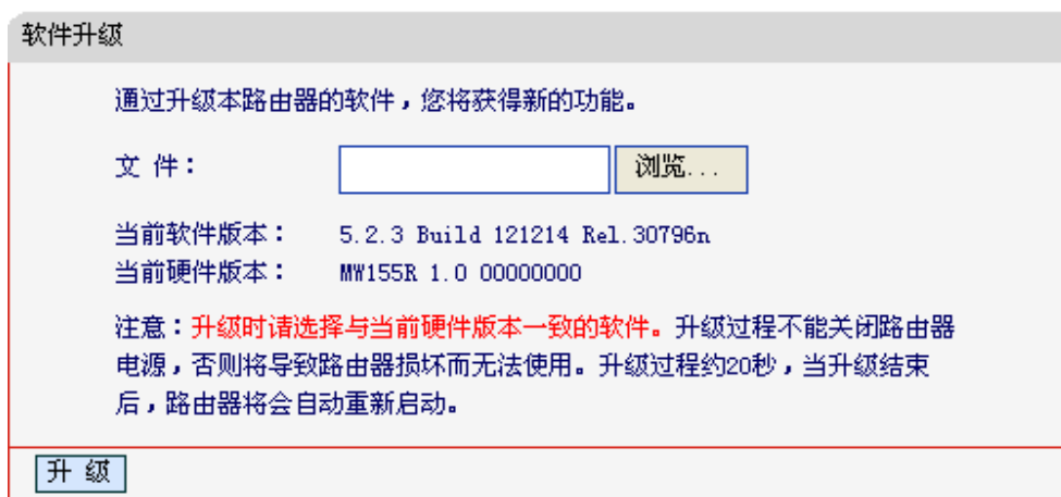
图 4-64 软件升级
