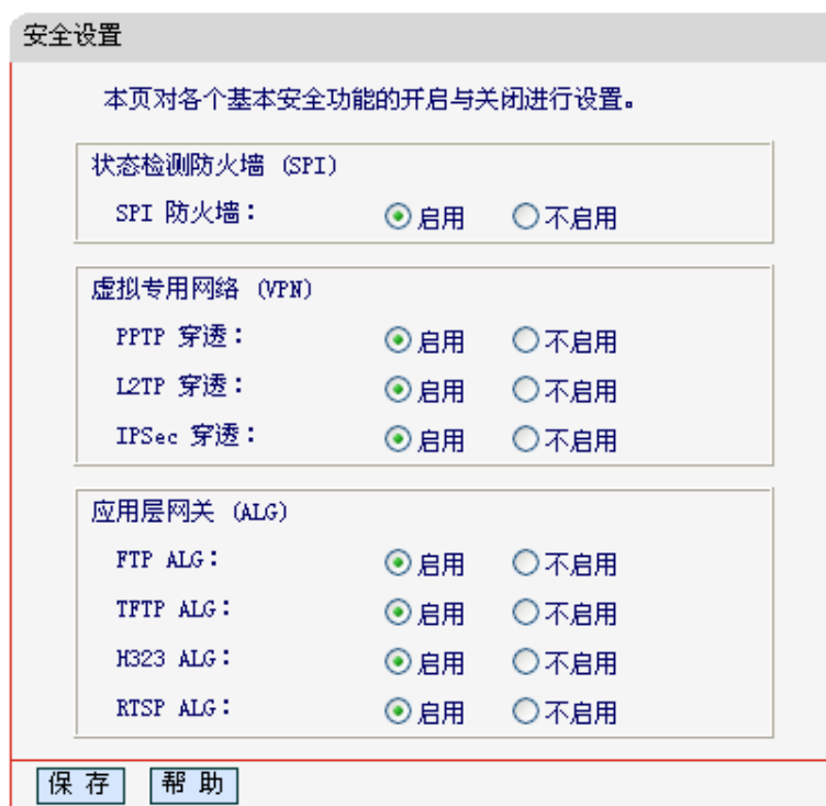
图 4-29 安全设置
