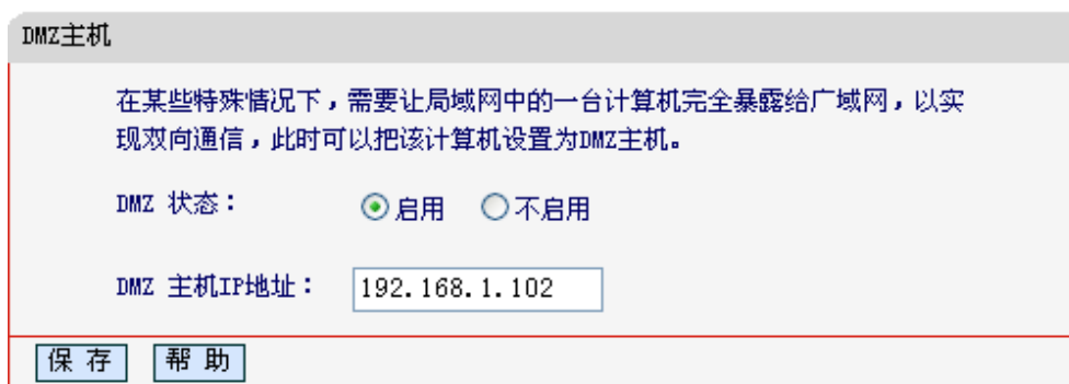
图 4-27 DMZ 主机
