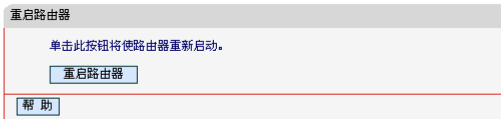
图 4-69 重启路由器
