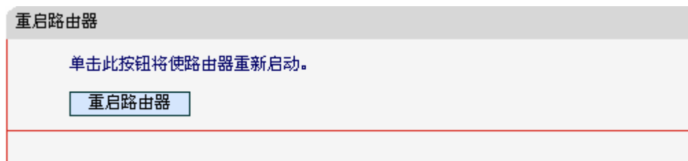
图 31 重启路由器
