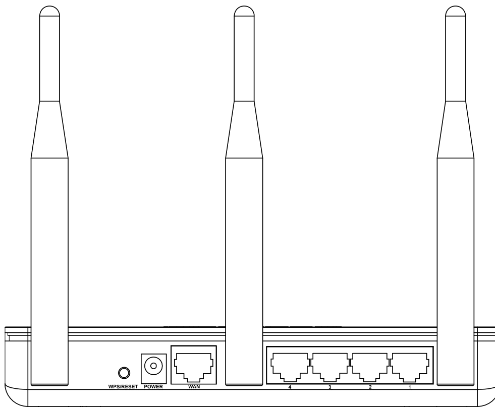
图 2-2 MW310R 后面板示意图
