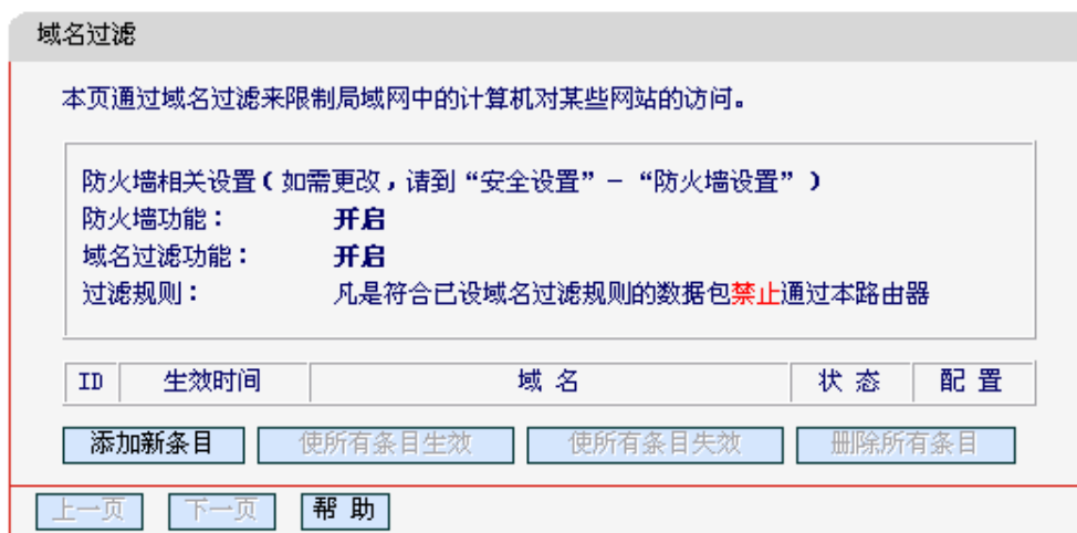
图 4-35 域名过滤
