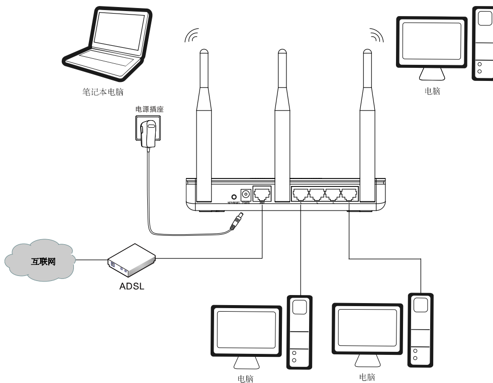
图 2-3 MW310R 硬件安装示意图
