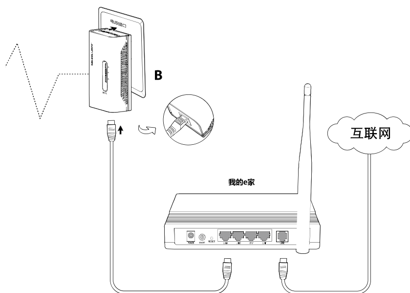
图2-4 网络连接图
