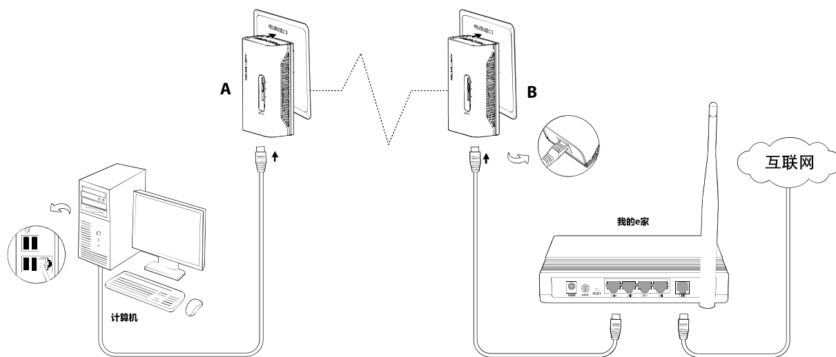
图2-5 整体连接图
