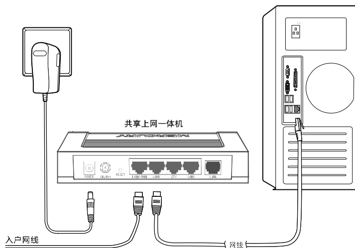
图4硬件连接图
