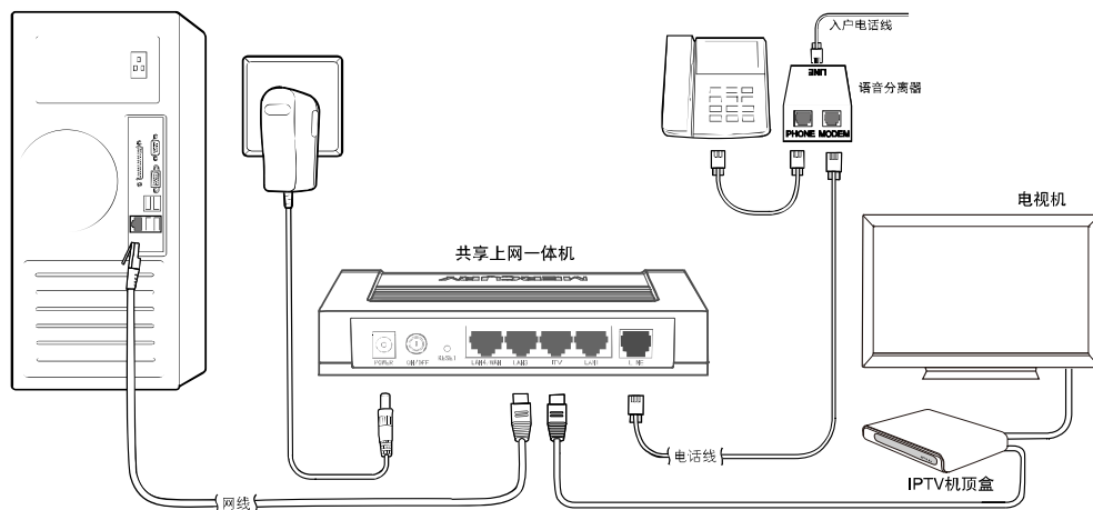
图3 硬件连接图
