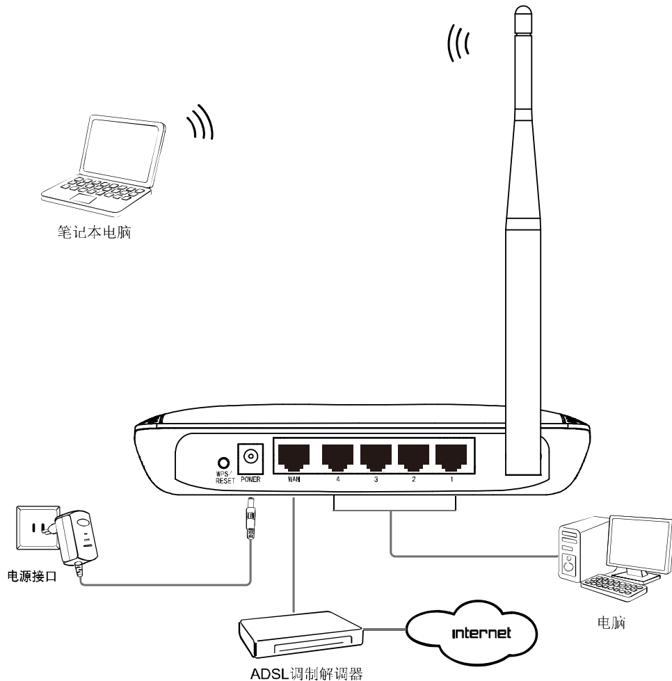
图 3 硬件连接图
