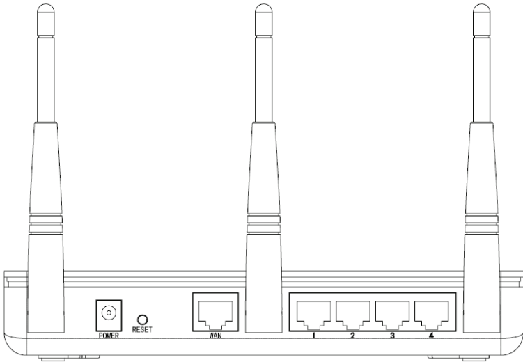
图 2 MWR300T+后面板示意图
