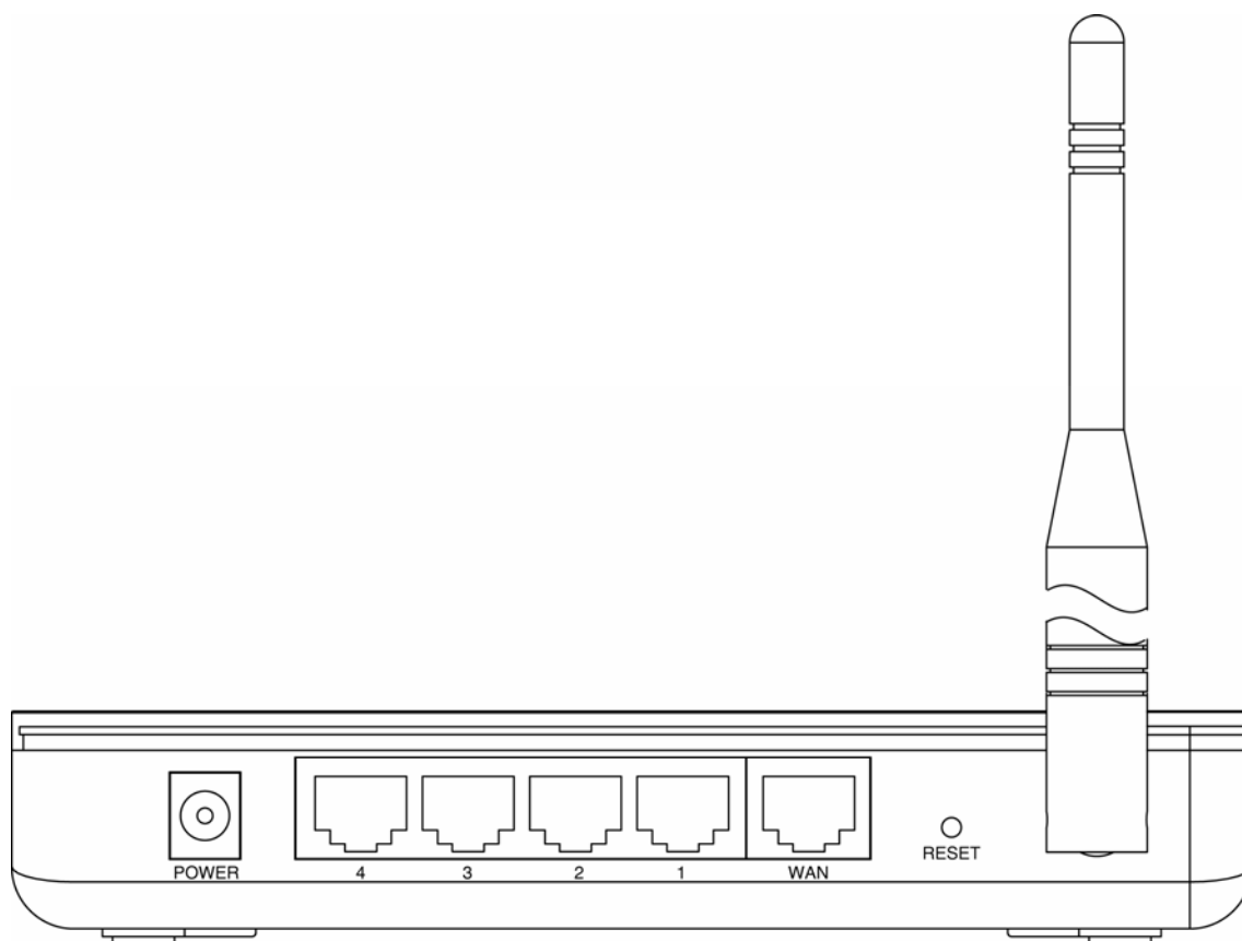
图 2 MW54R+后面板示意图
