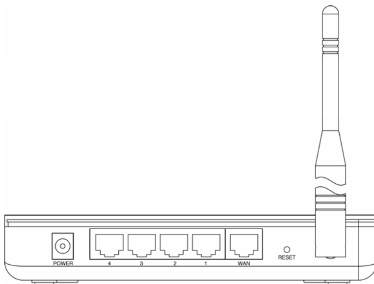
图 2-2 MW108R 后面板示意图
