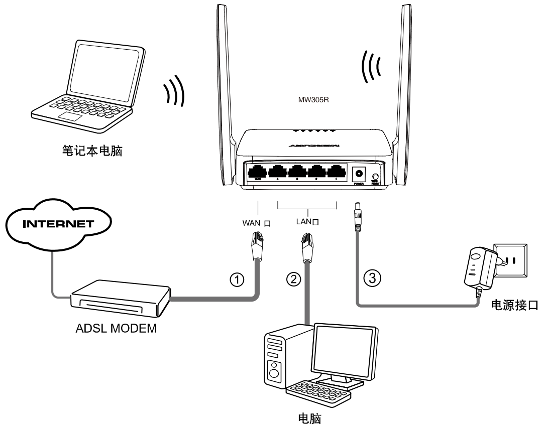
图 3 硬件连接图
