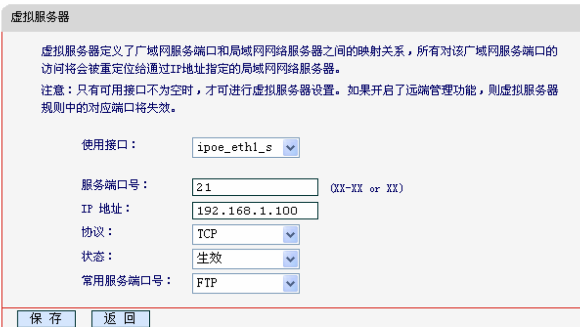
图 40 添加虚拟服务条目
